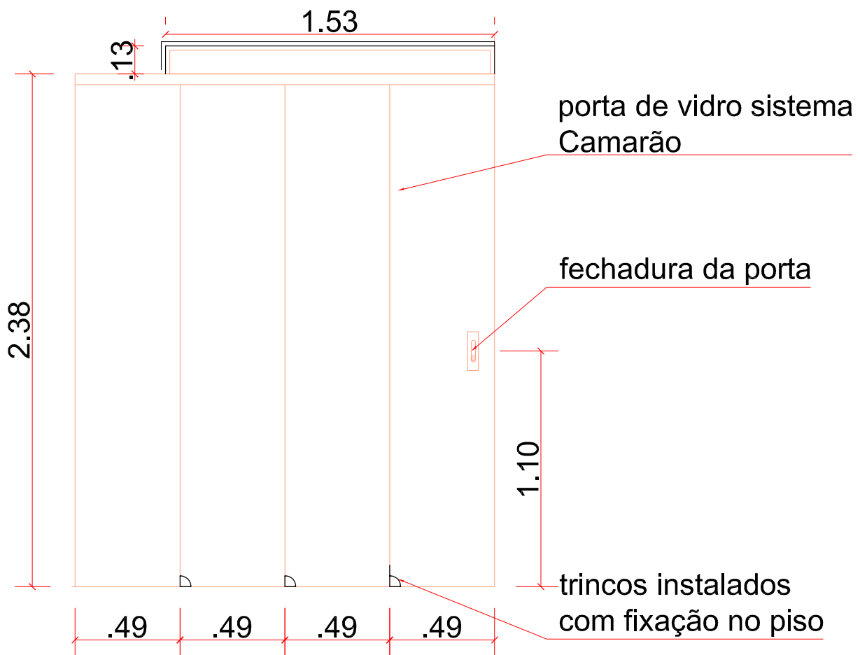
Vista Frontal - detalhamento porta
