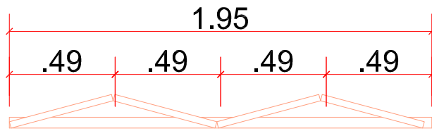
Planta Baixa - detalhamento porta
