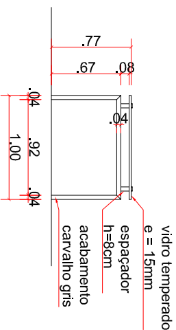
Vista Frontal - Aparador ESC.: 1/50
