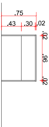
Vista Frontal - bancada computadores ESC.: 1/50
