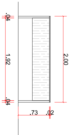
Vista 4 ESC.: 1/50
