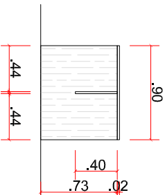
Corte BB ESC.: 1/50
