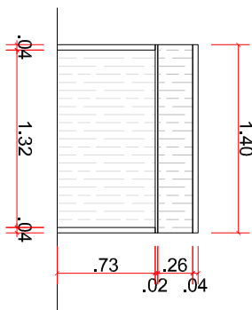
Vista 6 ESC.: 1/50
