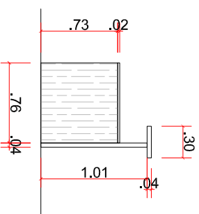
Vista 9 ESC.: 1/50
